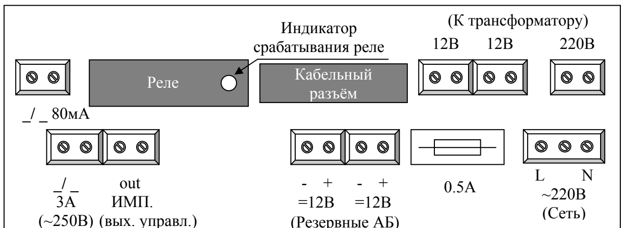
Рис. 3. Схема расположения разъёмов на монтажной плате модулей первичных часов СБЧС (две монтажных платы в каждом блоке).
