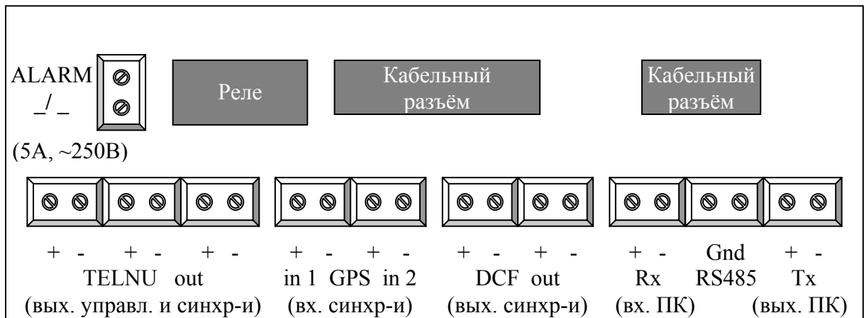
Рис. 2. Схема расположения разъёмов на монтажной плате модуля переключения и синхронизации СБЧС.
